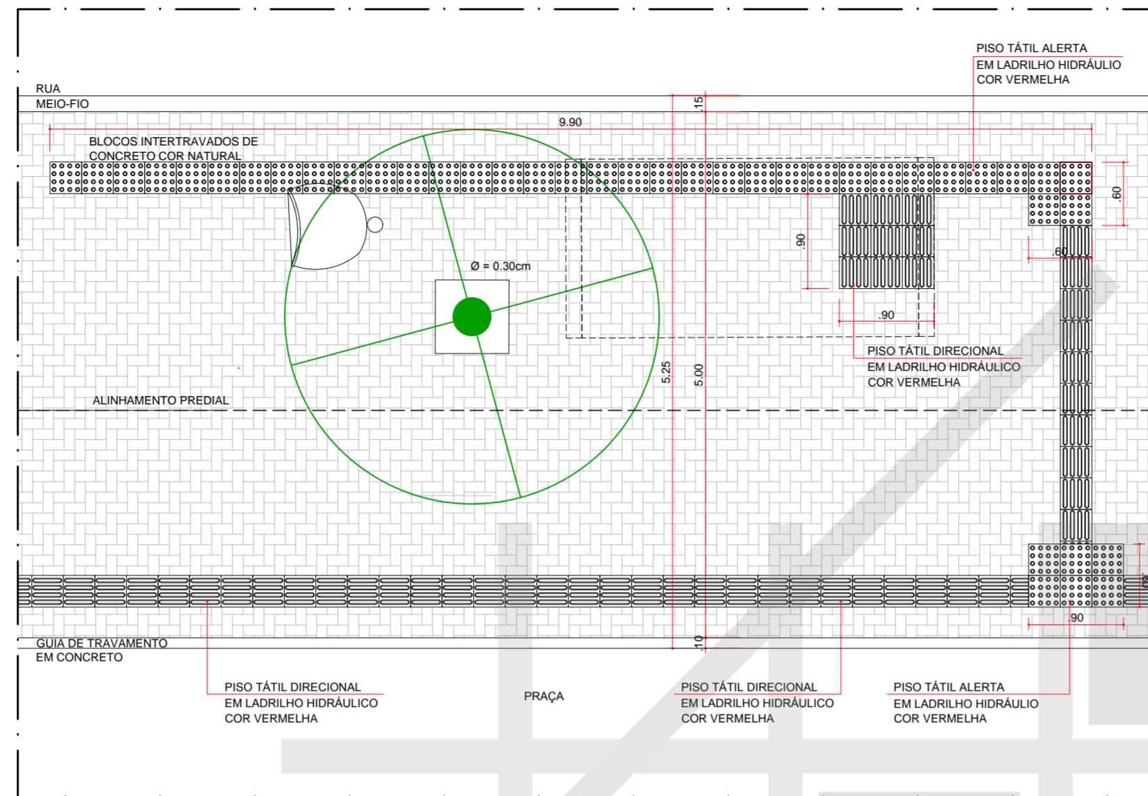
3 DET. 02 - PASSEIO 4.20m SINALIZAÇÃO TÁTIL NO PONTO DE ÔNIBUS ESCALA 1:50
