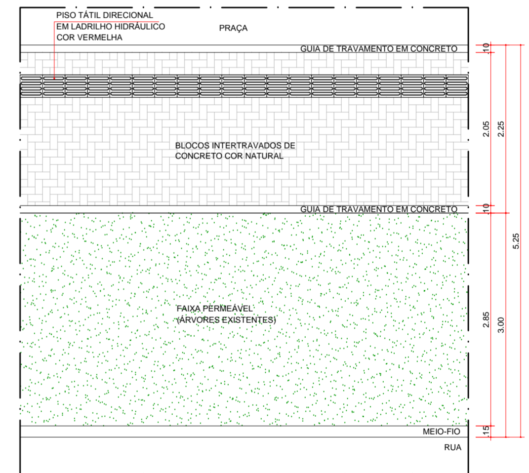
9 DET. 08 - PASSEIO 5,25m COM FAIXA PERMEÁVEL ESCALA 1:50
