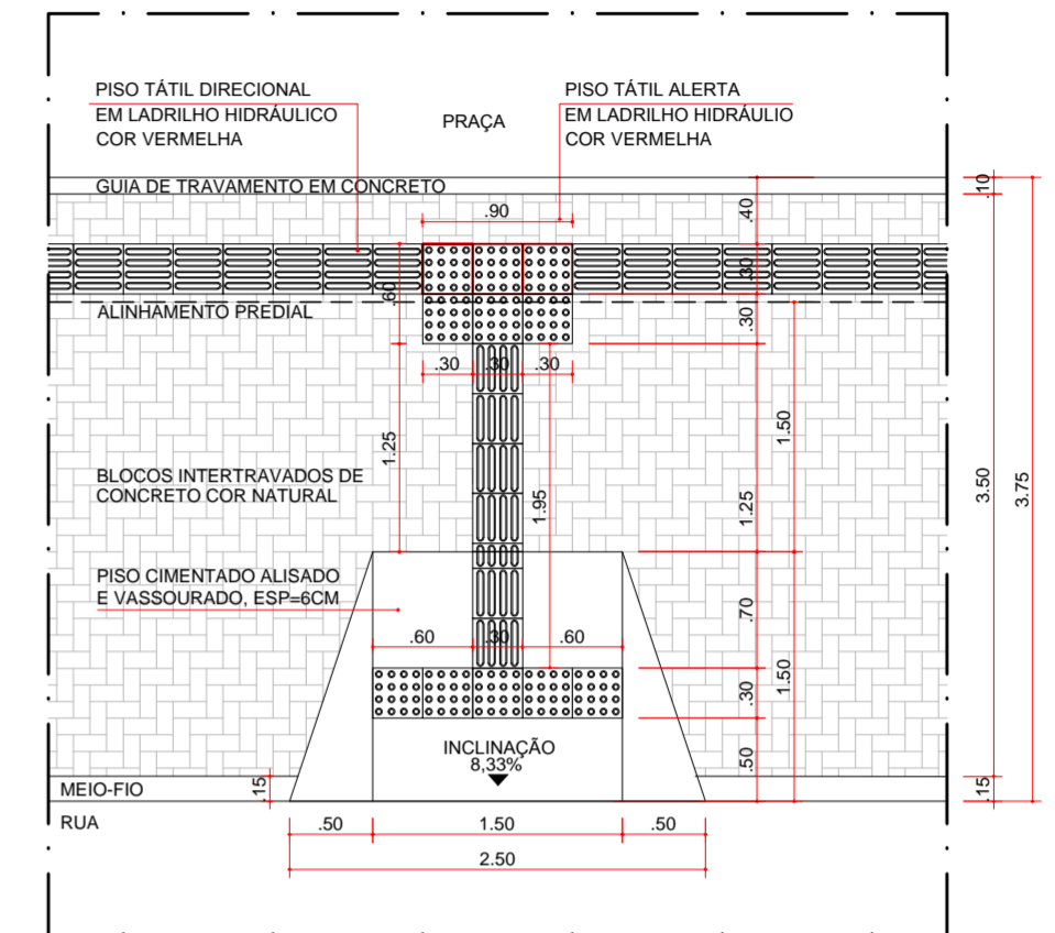
5 DET. 04 - REBAIXO DE GUIA PARA P.N.E. PASSEIO 3,75m ESCALA 1:50
