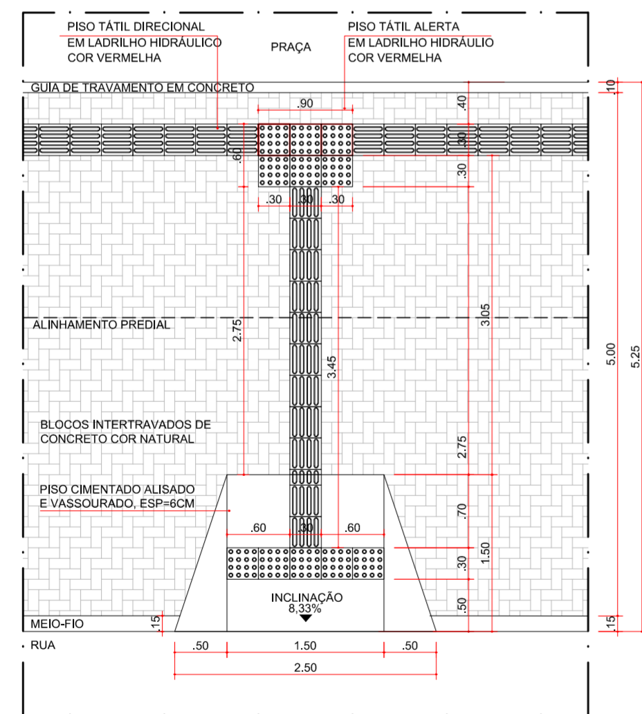
6 DET. 05 - REBAIXO DE GUIA PARA P.N.E. PASSEIO 5,25m ESCALA 1:50
