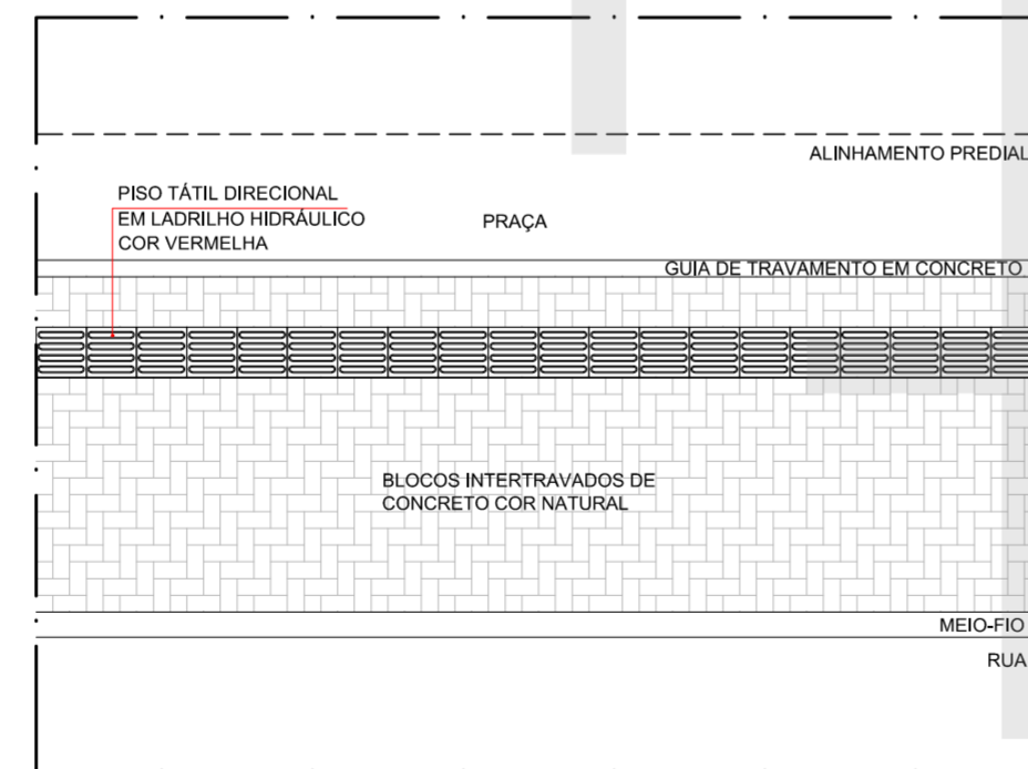
7 DET. 06 - PASSEIO 2,25m ESCALA 1:50
