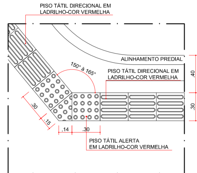
2 DET. 01 - PISO TÁTIL ALERTA ESCALA 1:25
