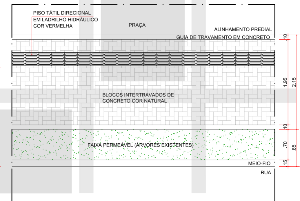
8 DET. 07 - PASSEIO 3,00m COM FAIXA PERMEÁVEL ESCALA 1:50
