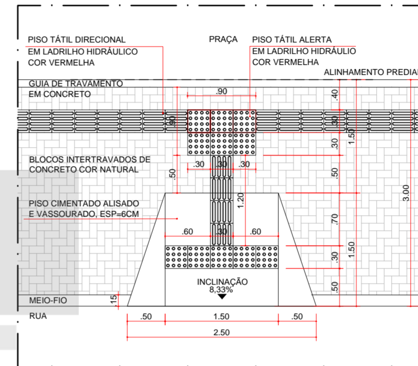
4 DET. 03 - REBAIXO DE GUIA PARA P.N.E. PASSEIO 3,00m ESCALA 1:50
