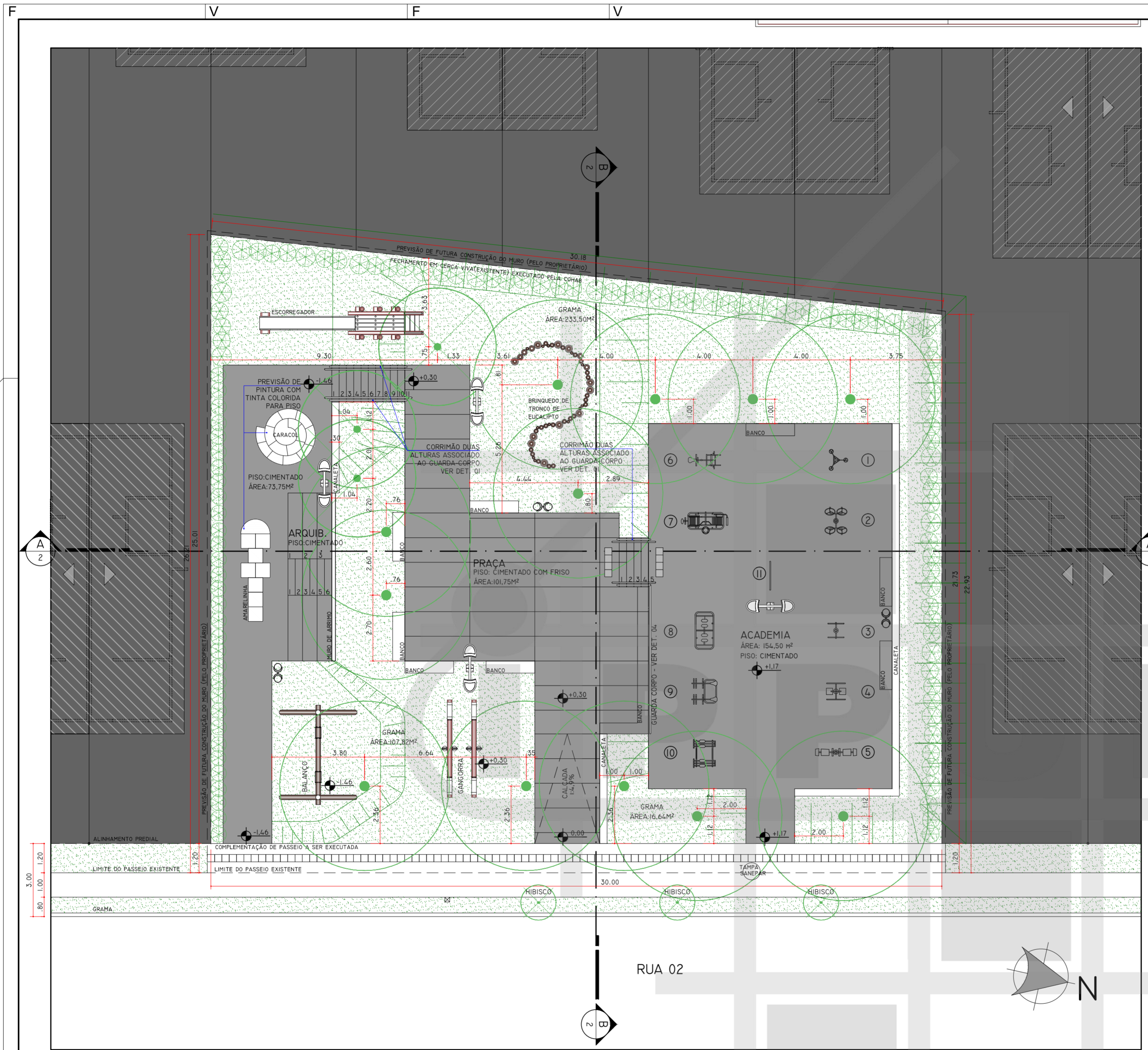
13 PLANTA PAISAGISMO - PRAÇA 05 ESCALA 1:125
