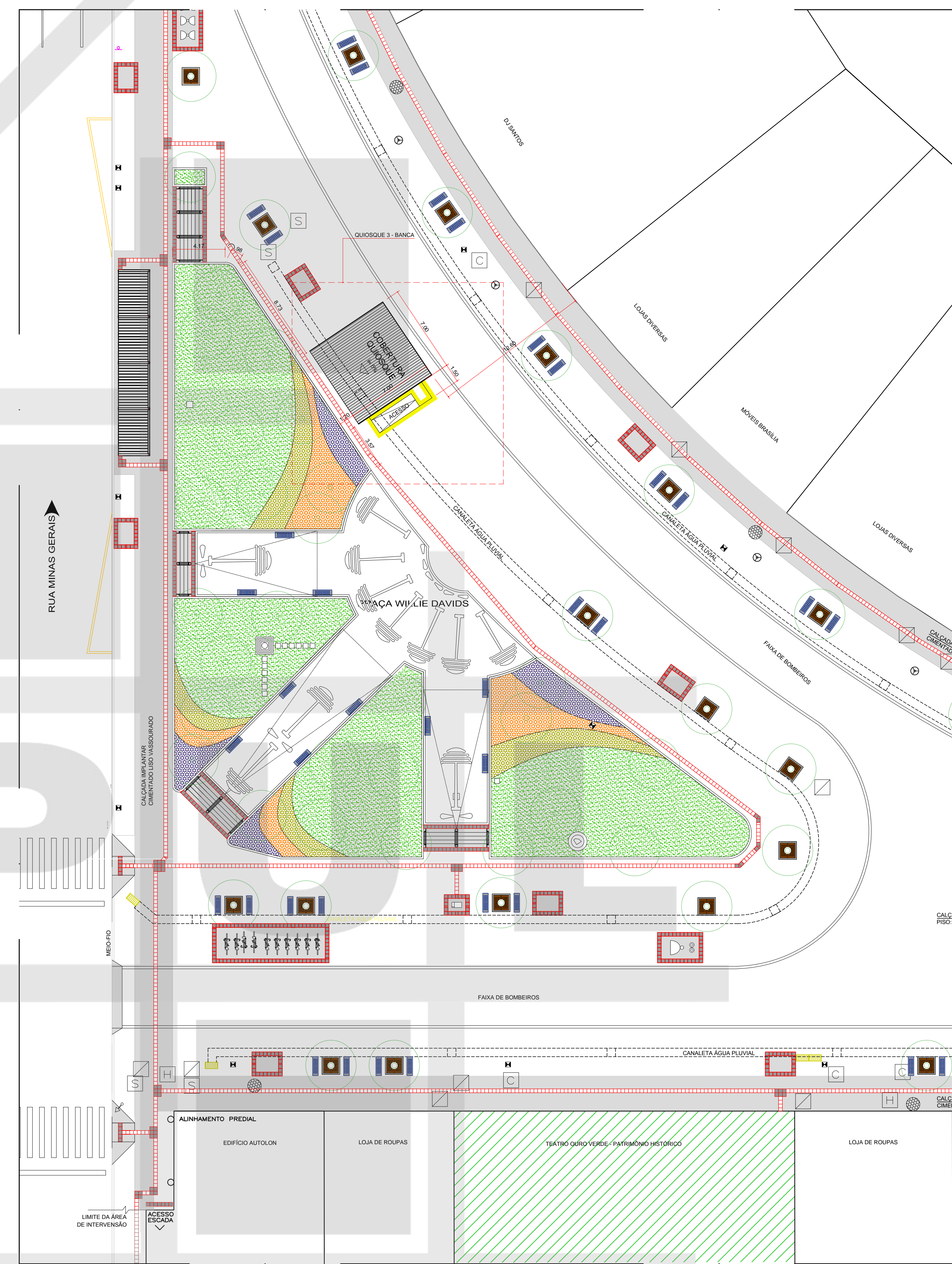
2 IMPLANTAÇÃO - PROJETO REVITALIZAÇÃO CALÇADÃO - QUIOSQUE 3 ESCALA 1:200
