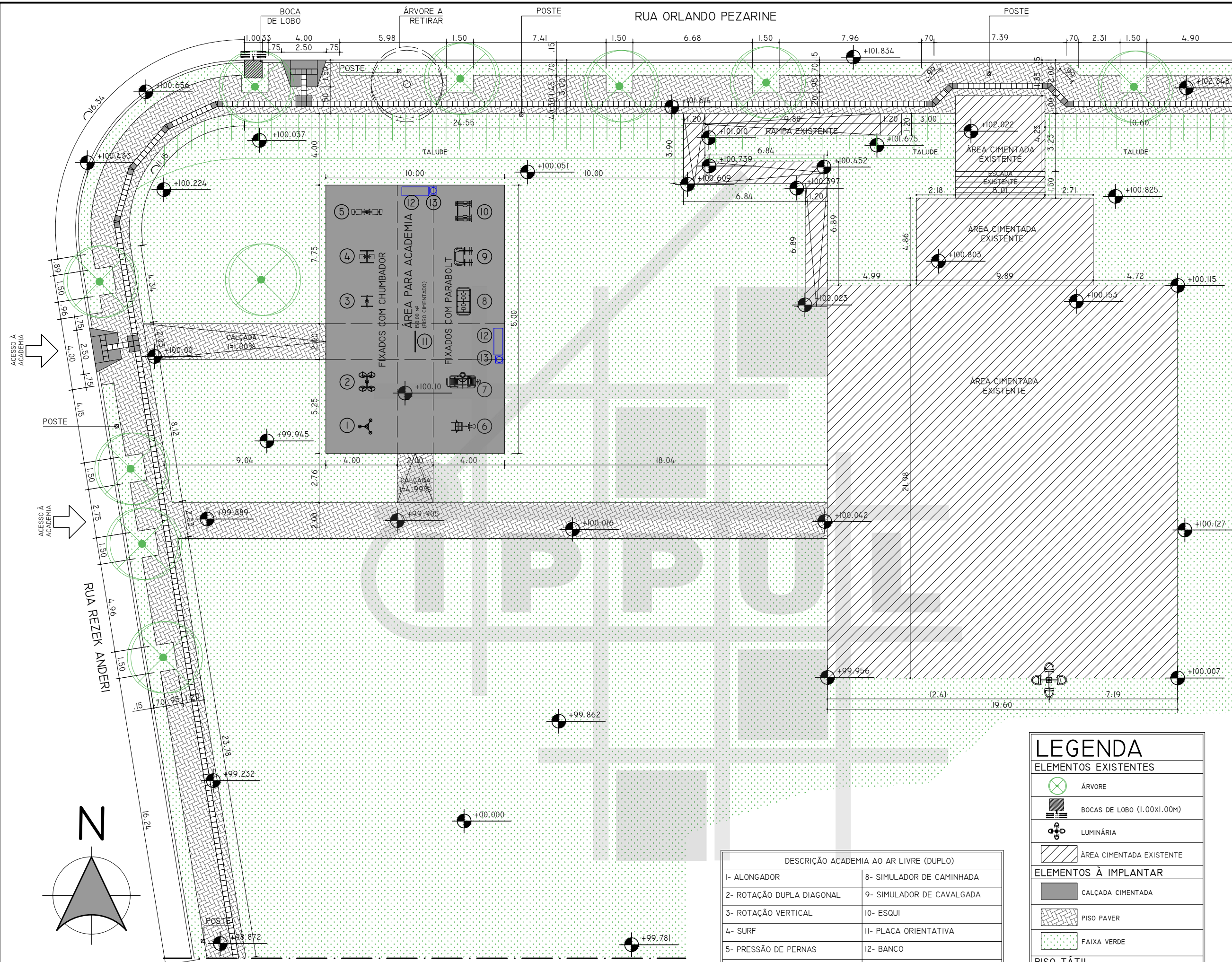
8 IMPLANTAÇÃO DE ACADEMIA ESCALA 1:200
