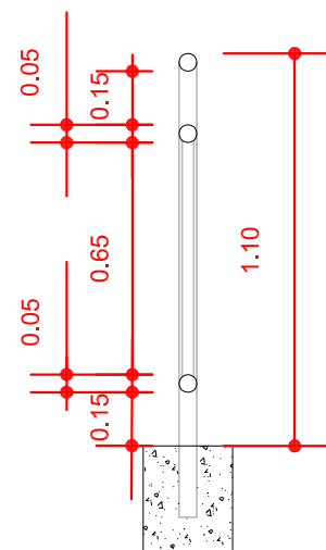
CORTE
