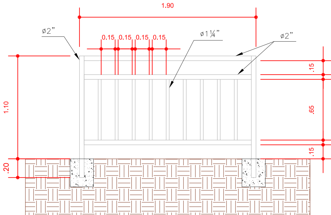
ELEVAÇÃO
